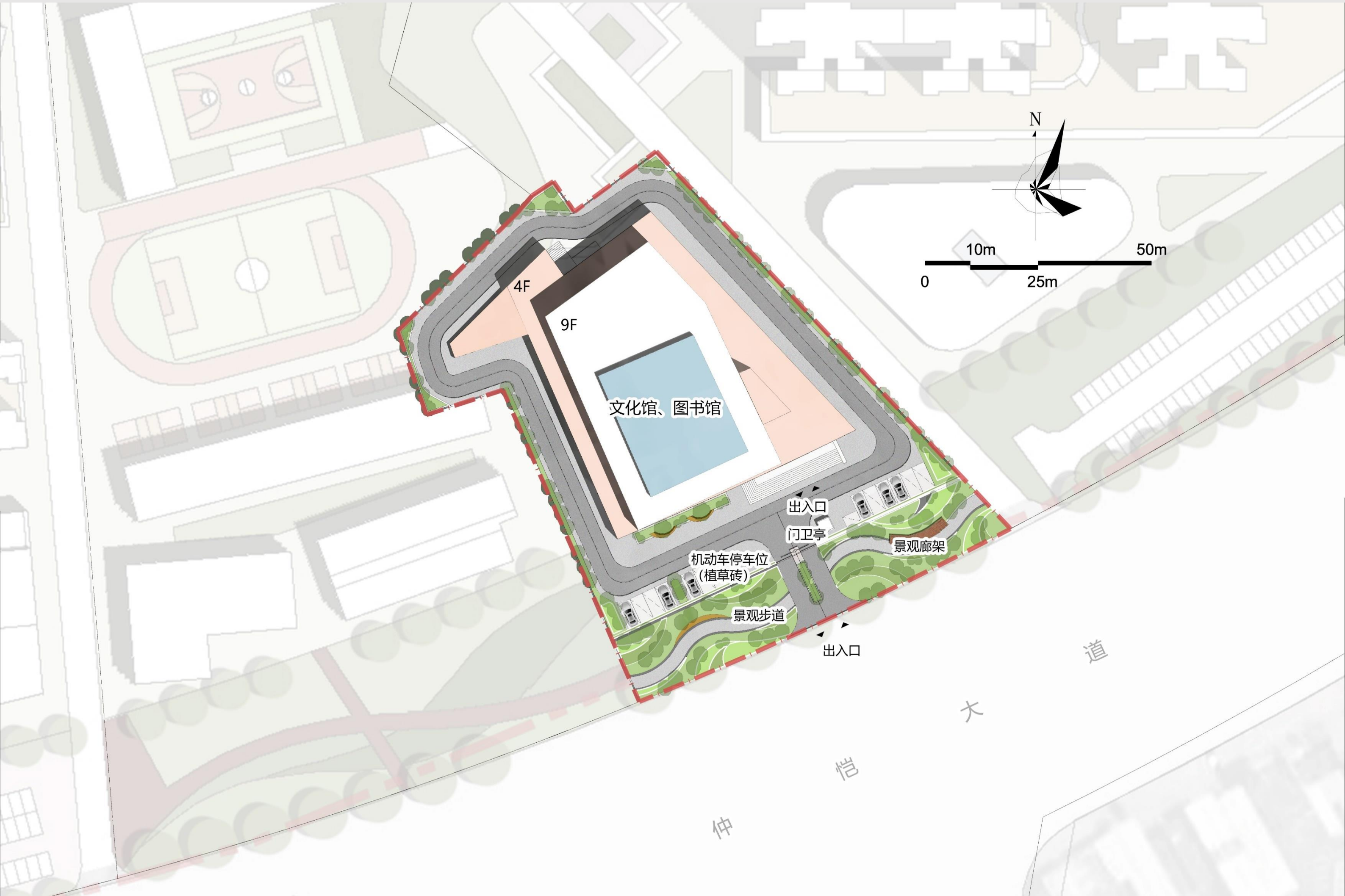
规划平面图
